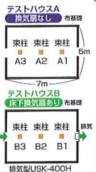
含水率 (%) 《当社テストハウスにおける床下束柱木材含水率比較》
