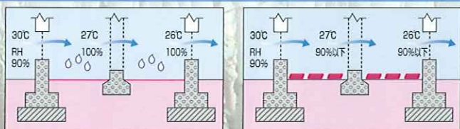
防湿フィルム・コンクリートによる結露 「New炭一郎」敷込みによる結露改善 ※上記比較は、当社参考データによるシミュレーションです。
