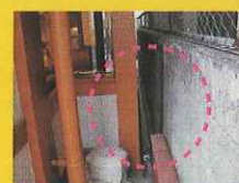
店舗基礎コンクリートの破損穴U字側溝から穴に入る。
